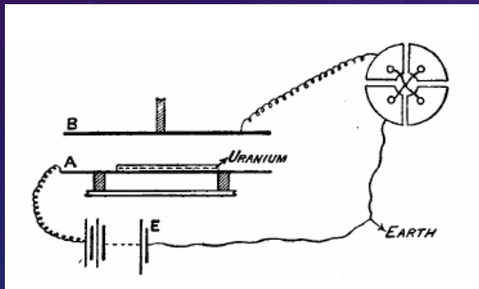
Квадрантни електрометар
