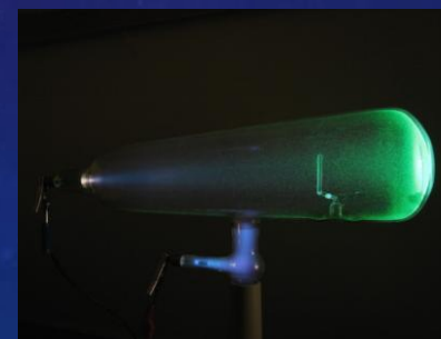
Crookes-ова цев
