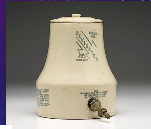
Радијумска вода
